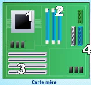
Carte mère
